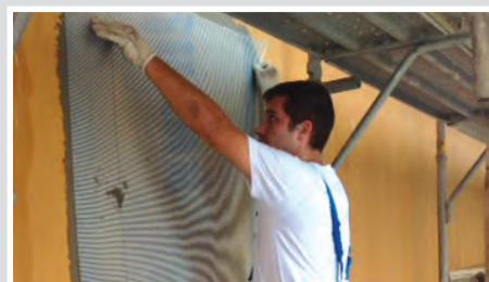
Stesura della rete di armatura
